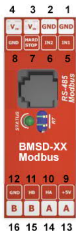
Рис. 2. Схема расположения и назначение клемм и элементов управления
